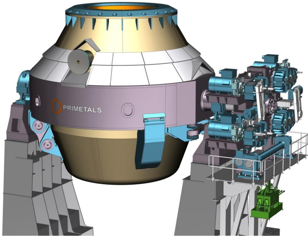
俄罗斯梅切爾集團車里雅賓斯克冶金廠（ChMK）煉鋼車間新轉爐的計算機效果圖
