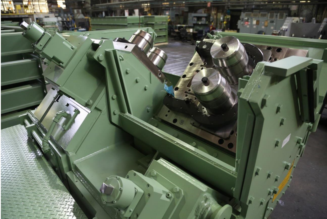
Primetals Technologies の高速線材圧延機用超剛性 (UHD) 圧延ユニット
