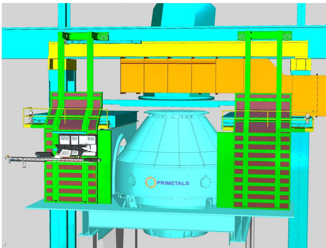
Computeranimierte Darstellung des LD(BOF)-Konverters von Primetals Technologies für ArcelorMittal Ruhrort
