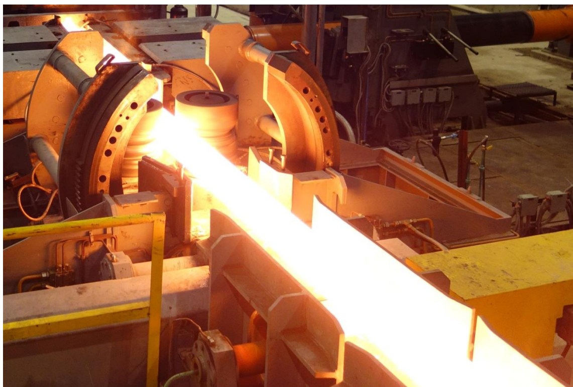
Primetals Technologies の特殊形鋼圧延プラント用の自動棒鋼搬送装置 (設置例)
