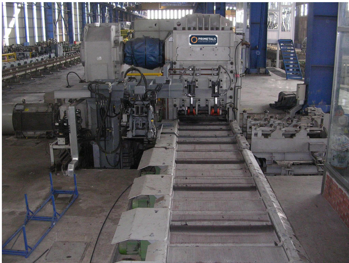
Ножницы холодной резки и рольганг для сортопрокатного стана от Primetals Technologies
