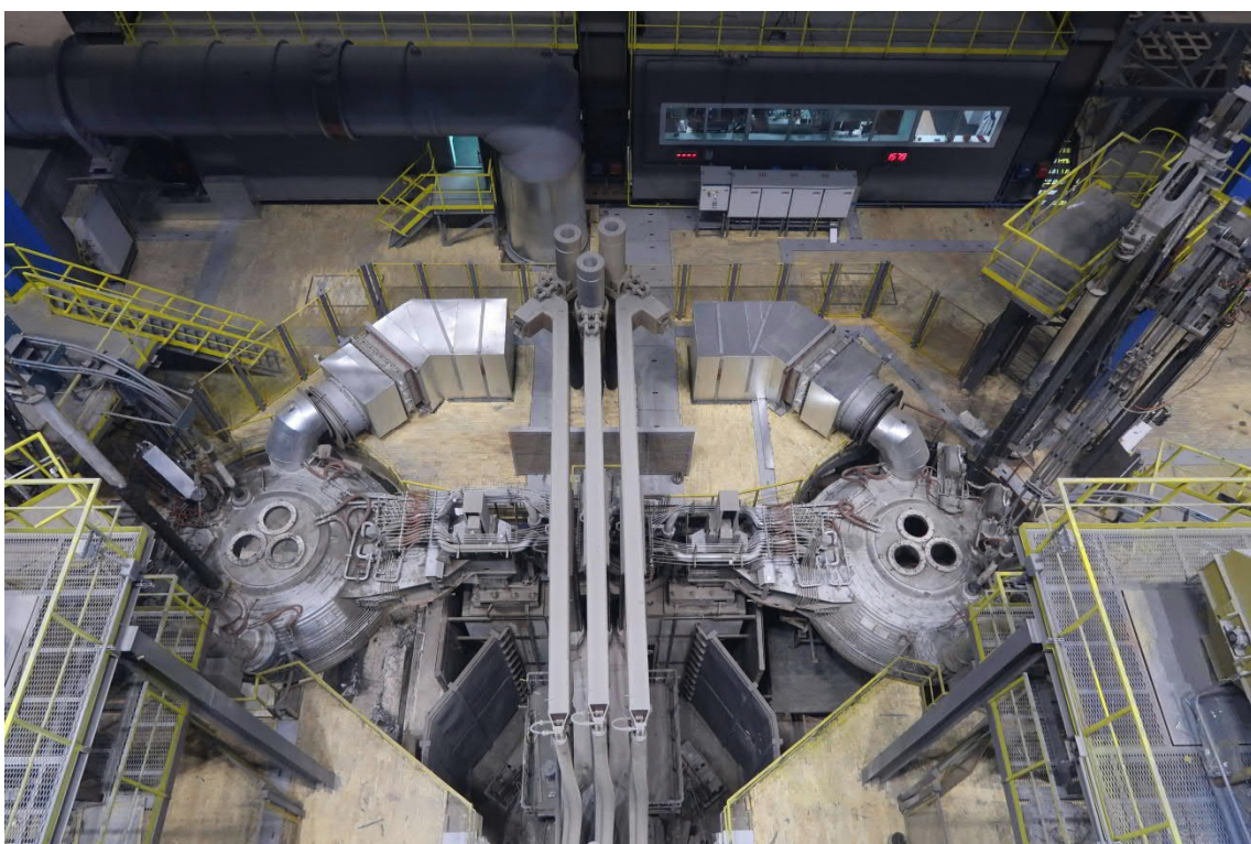
Двухпозиционная установка «печь-ковш», поставленная Primetals Technologies в ККЦ ЧерМК в г.Череповец, ПАО «Северсталь».
