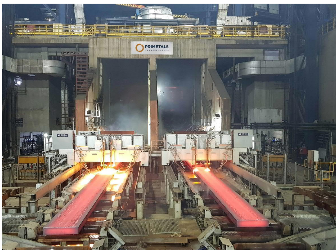
インドの JSW スチール社ドルビー工場に納入されたスラブプライメタルズテクノロジー製連鑄機
