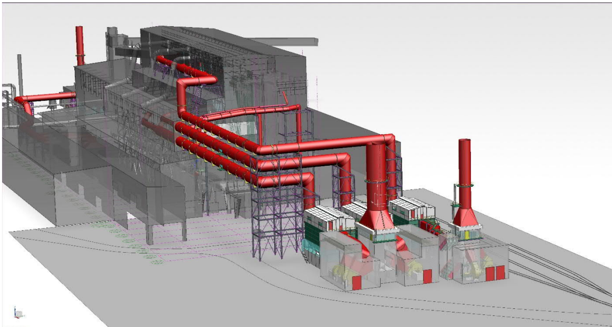
3-D изображение системы вторичного обеспыливания Primetals Technologies для ММК (Россия).
