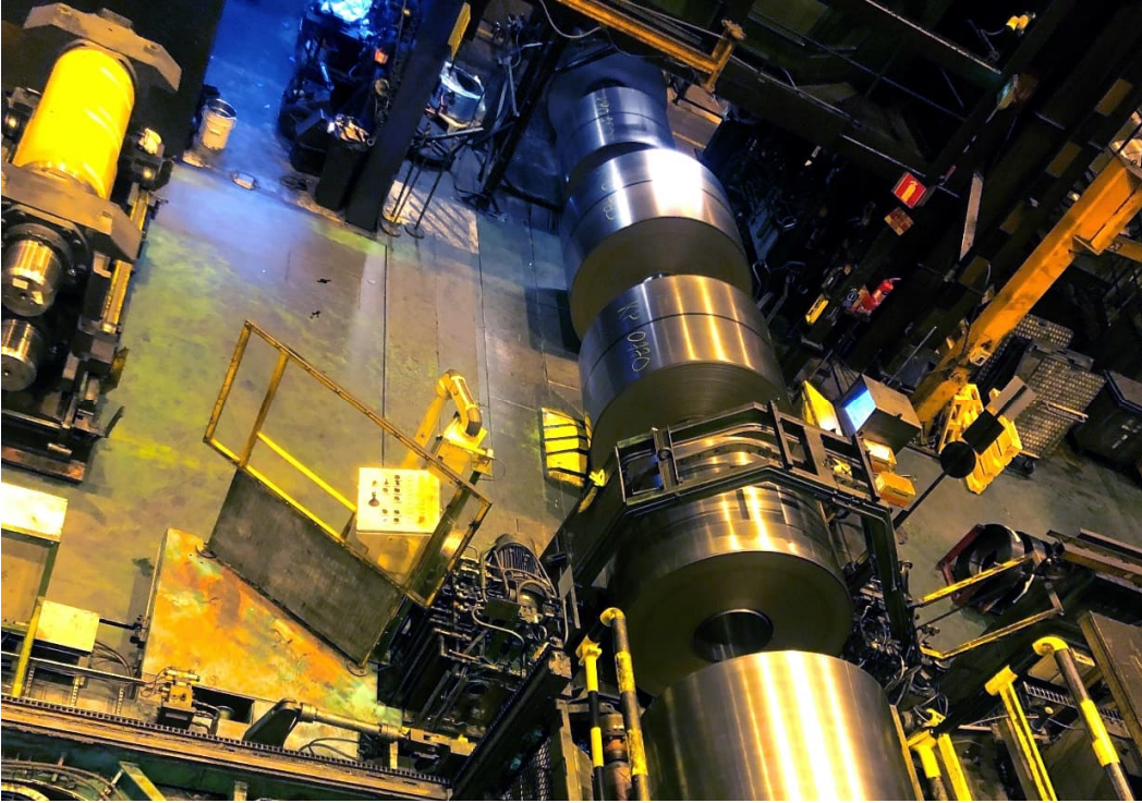
SSAB ハメーンリナ製鉄所のミルスタンド更新工事フェーズ 1 完工後のファーストコイル
